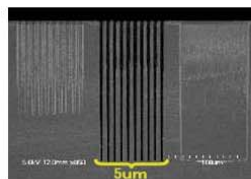
深溝加工 (幅:5µm, 深さ:200µm)
