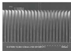
深溝加工 (幅:20µm, 深さ:400µm)
