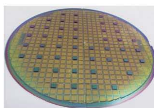
8" TSVウェハへのチップ接合実装例
