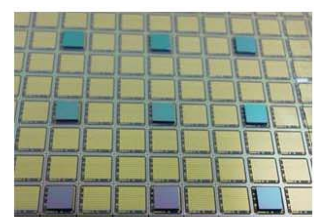
接合実装チップ拡大写真
