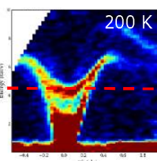
中性子非弾性散乱のフォノン光学モードのソフトニングの観察
