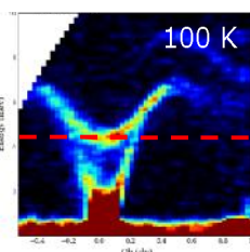
中性子非弾性散乱のフォノン光学モードのソフトニングの観察
