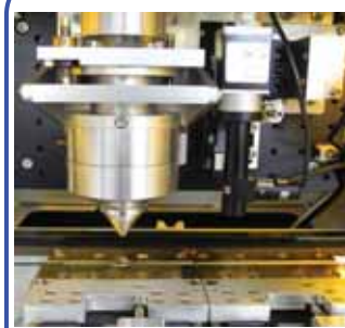
レーザースクライブ装置
