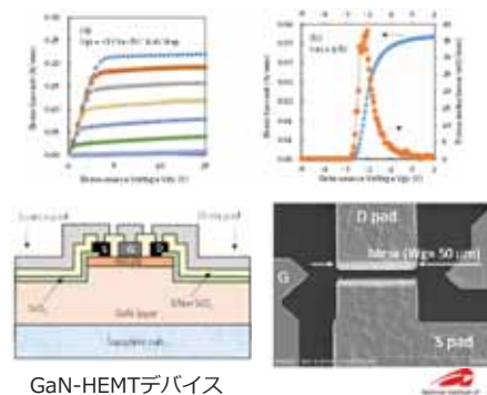
GaN-HEMTデバイス
